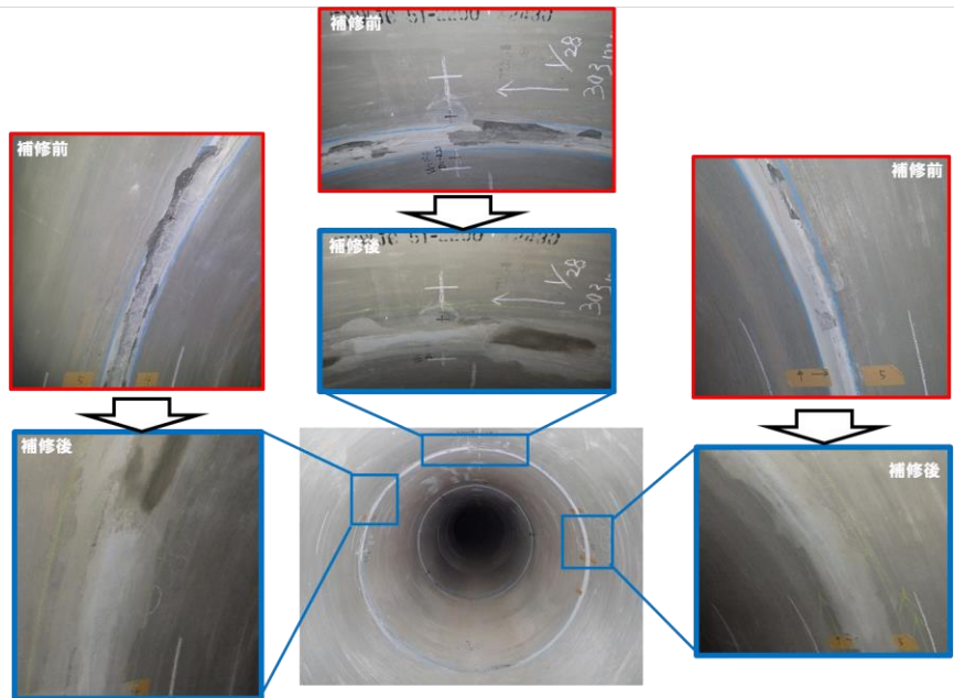
管渠の目地モルタルの補修状況 (写真)
