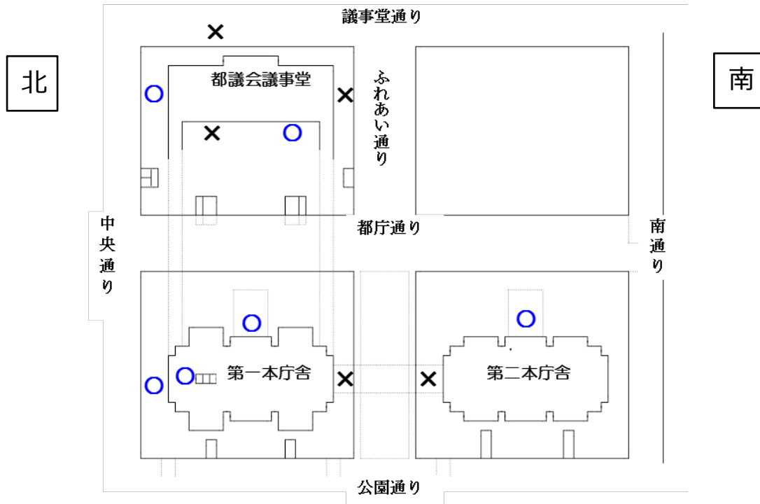
都本庁舎レイアウト図（1階）
