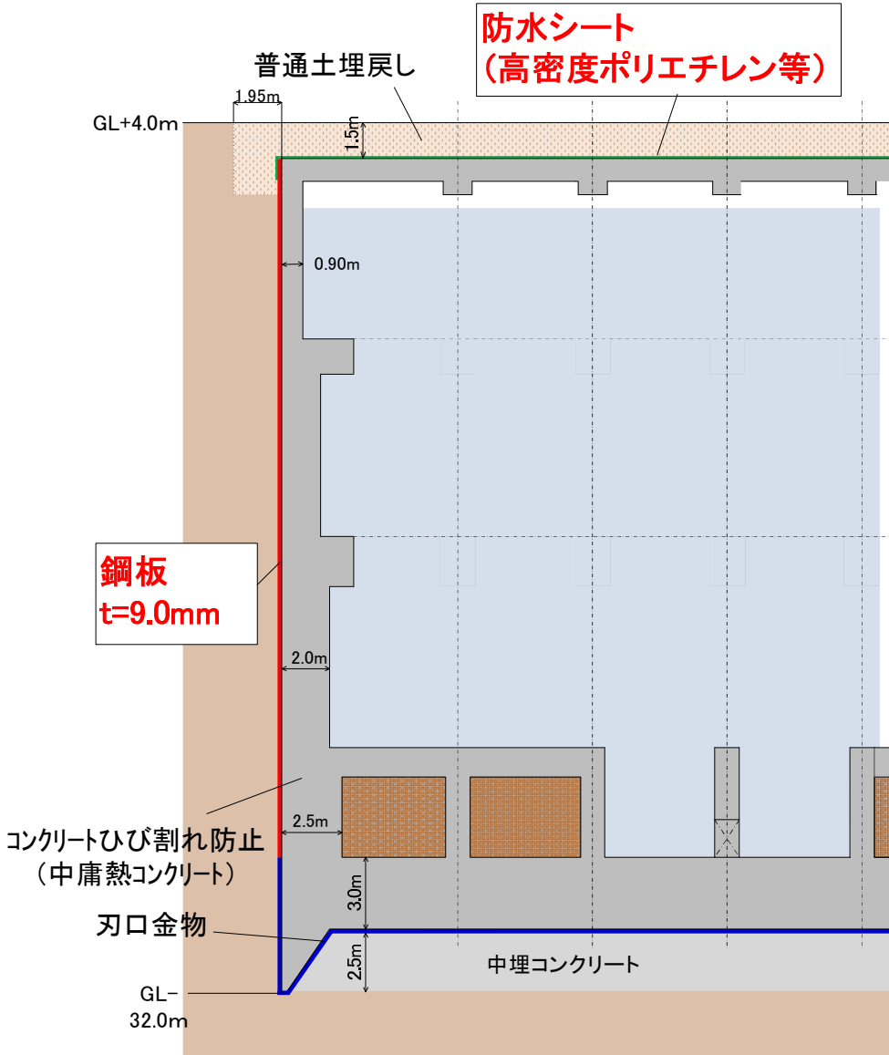
配水池断面図
